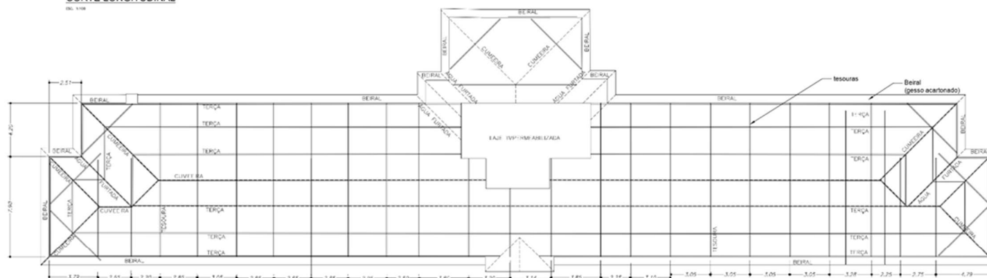
PLANTA COBERTURA - TESOURAS/ TERÇAS
