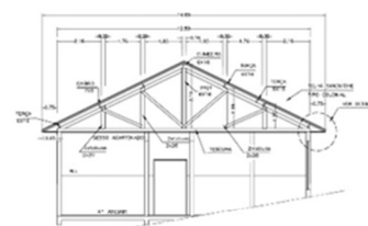
CORTE TRANSVERSAL
